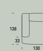
Elemento a isola Maxi SX-DX Deep seat el. Maxi LH - RH Elém. assise plus Maxi GA - DR Inselement Maxi LI - RE
