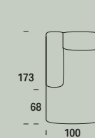
Chaise longue Midi SX-DX Midi chaise longue LH - RH Chaise longue Midi GA - DR Chaiselongue Midi LI - RE
